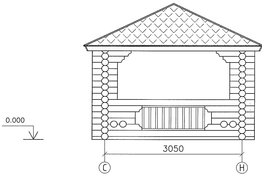
Aansicht - A
