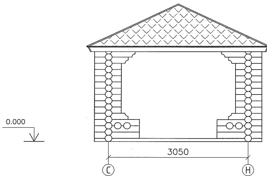
Ansicht - B
