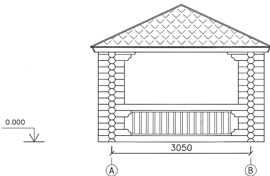
Ansicht - H
