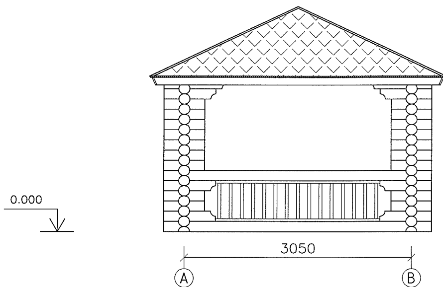
Ansicht - C
